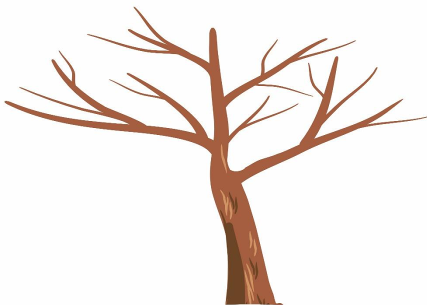
Рисунок 2. «Дерево безопасности»
